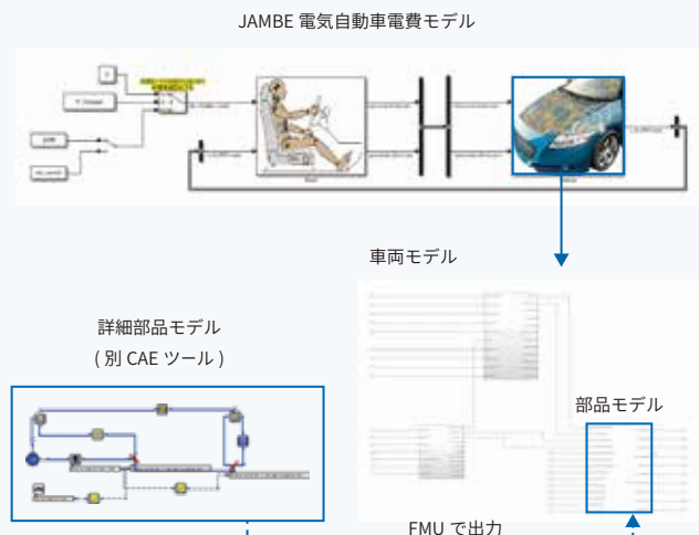
図：「自動車開発におけるプラントモデル I/F ガイドライン準拠モデル（電気自動車用電費モデル）解説書」より
